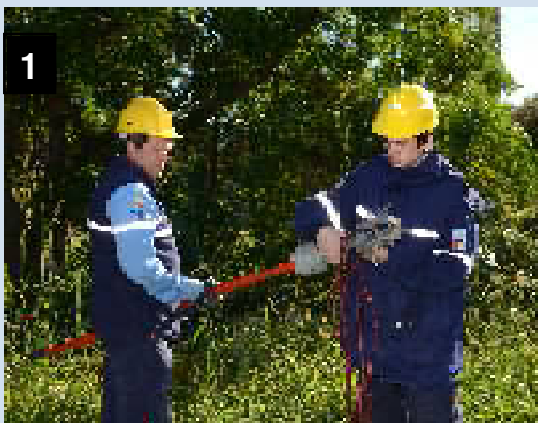
1. Verificación del buen contacto de los morsetos / 2. El carretel del cable de la puesta a tierra debe estar absolutamente desarrollado / 3. El cable debe estar separado del cuerpo del operario.
